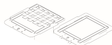
Seteplate med utsparing
