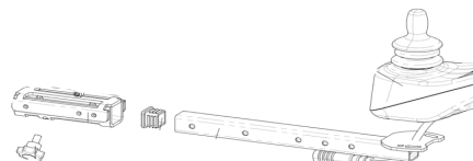
Feste Joystick fast med Quick release
