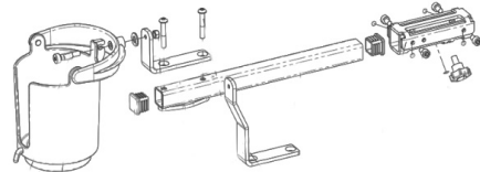
Holder kopp
