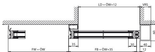
Horizontalsnitt 1-fløyet
