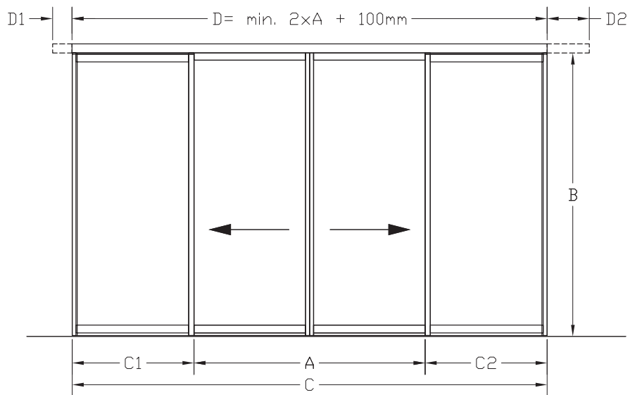
Konstruksjon – 2-fløyet med sideparti
