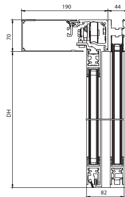
Loddrett snitt med bæreprfil og sideparti
