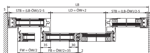
Horizontalsnitt med sidefelt
