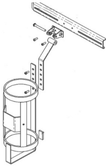
Holder oksygenflaske
